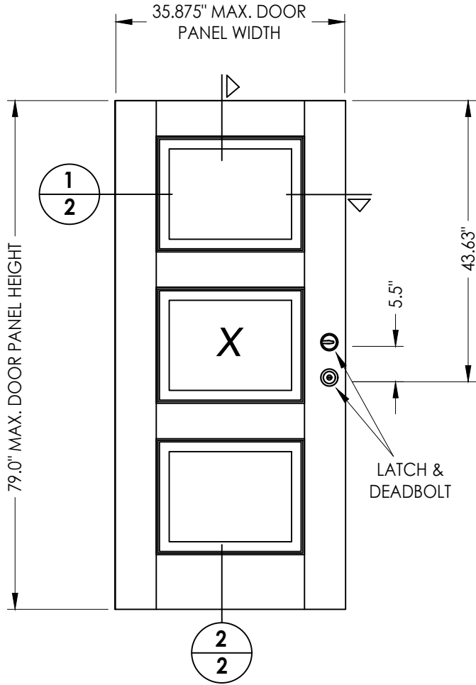
40 DOOR PANEL Mastergrain
